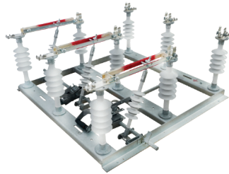
Silikon İzolatörlü Harici Tip Ayırıcı
