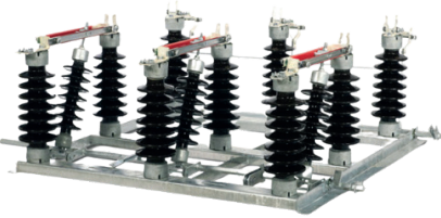
Porselen İzolatörlü Harici Tip Ayırıcı
